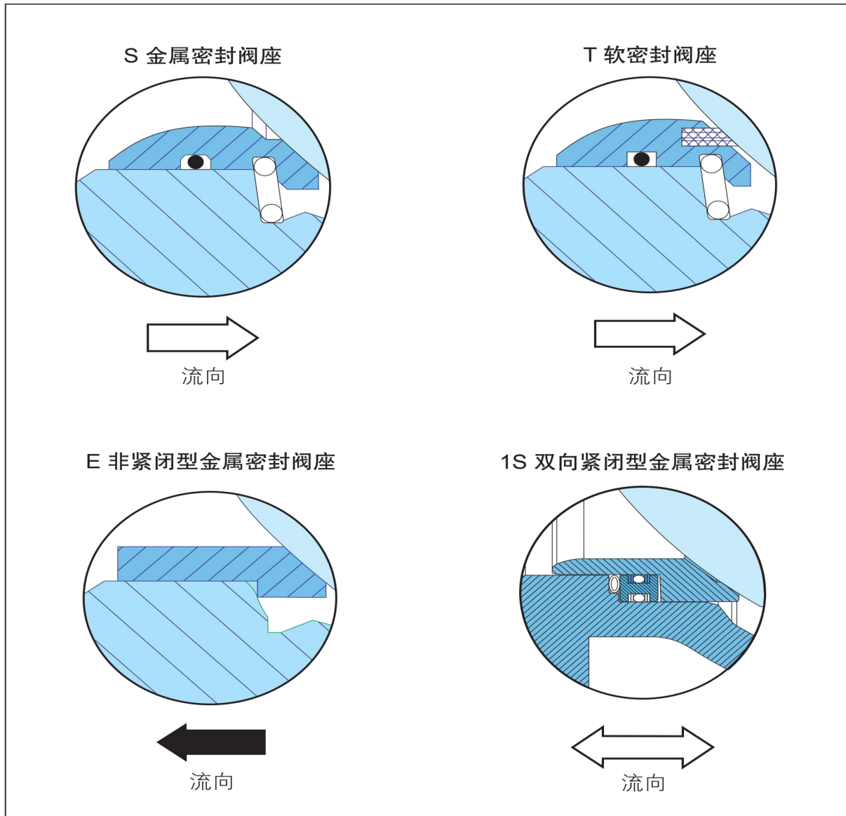
E非紧闭型金属密封阀座
